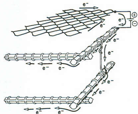
(Esquema de un Sistema de P C por Corriente impresa)
